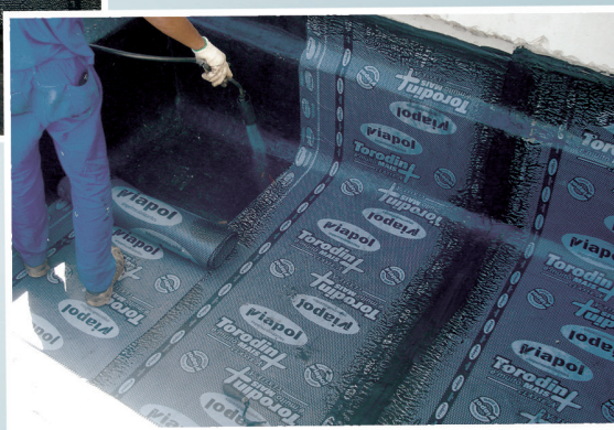
Colagem de manta asfáltica
